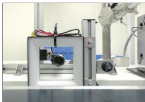
印字確認用カメラ1台
